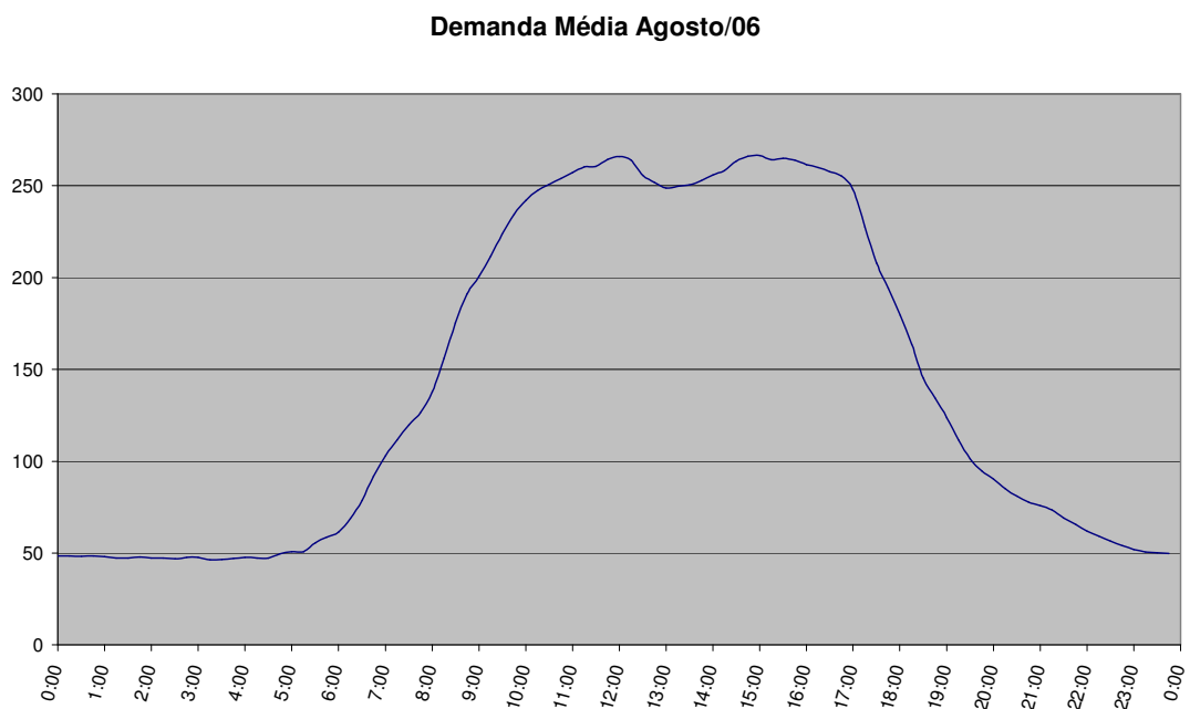
Figura A 8: Demanda média Agosto/2006
