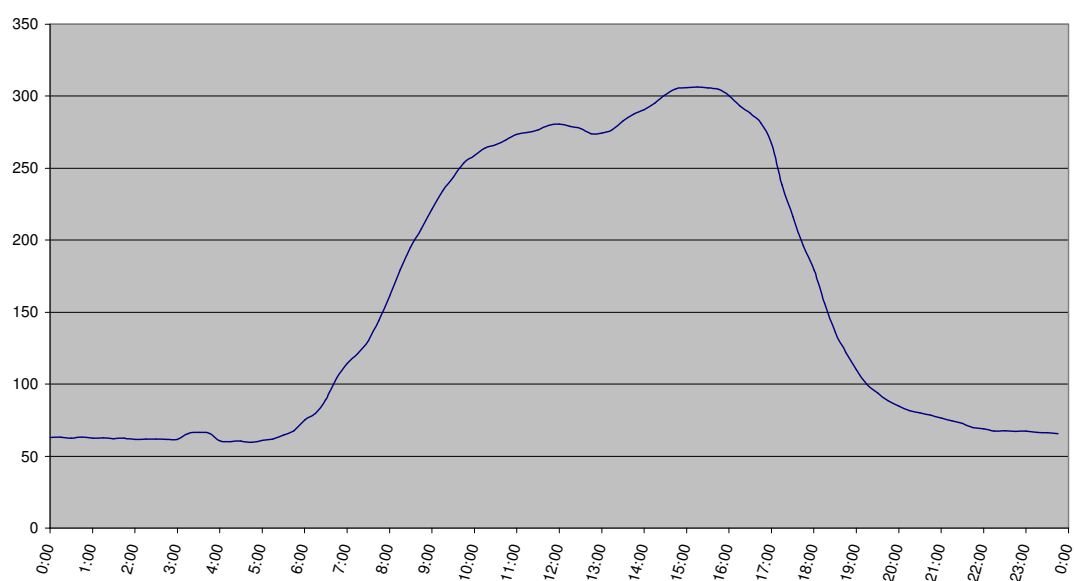
Figura A 2: Demanda média Fevereiro/2007
