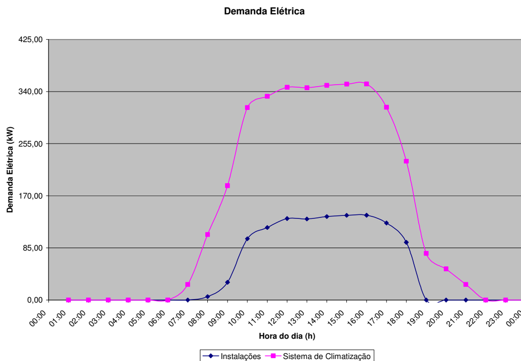
Figura 6.10 – Gráfico da demanda elétrica - dia típico de verão (proposta 4)
