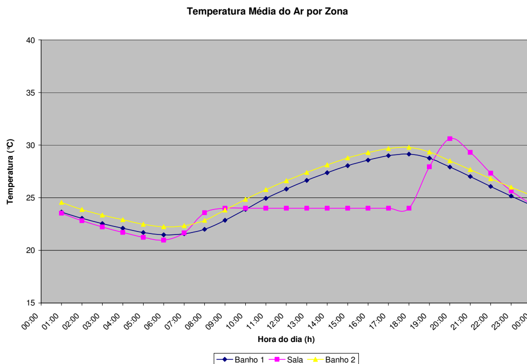
Figura 6.9 – Temperatura média do ar por zona (proposta 4)
