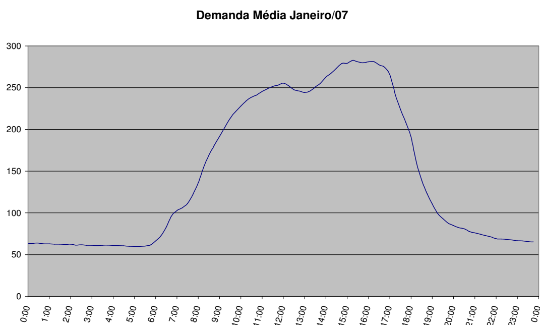
Figura A 1: Demanda média Janeiro/2007
