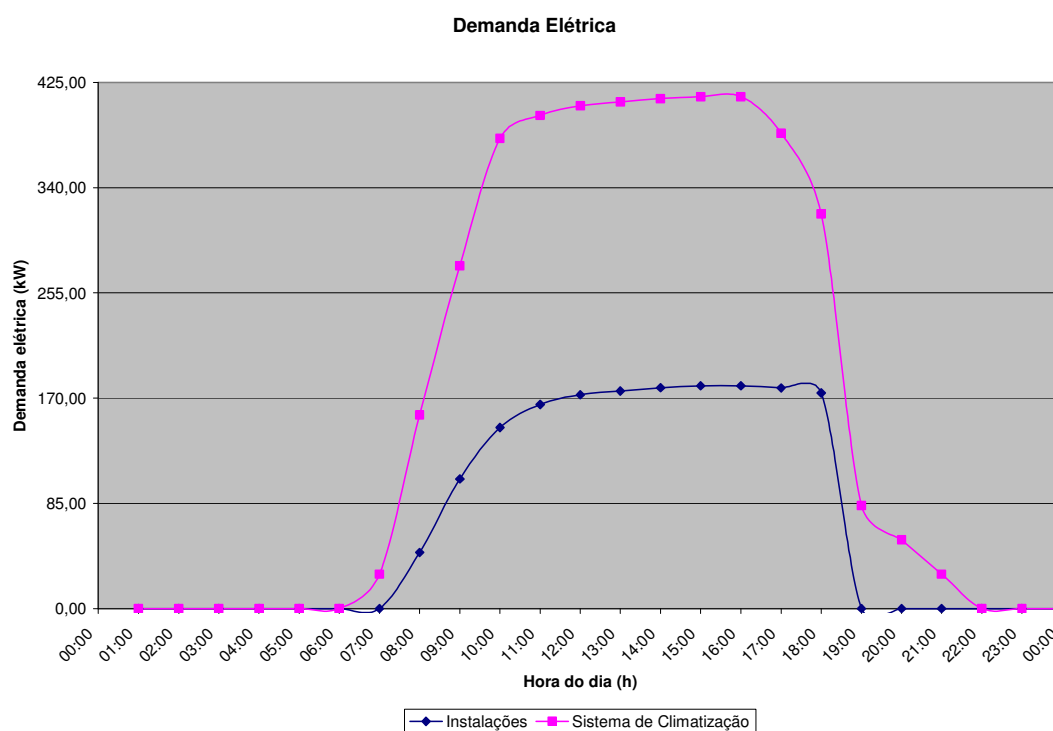
Figura 6.6 – Gráfico da demanda elétrica - dia típico de verão (proposta 2)
