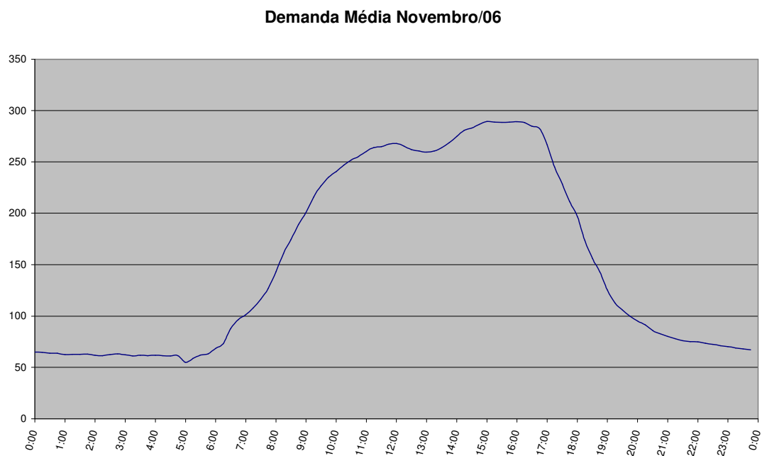
Figura A 11: Demanda média Novembro/2006
