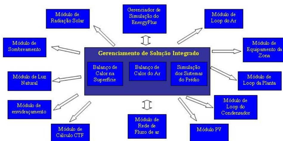
Figura 3.1 – Esquema do EnergyPlus
