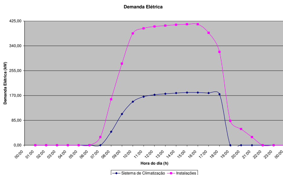
Figura 6.2 – Gráfico da demanda elétrica - dia típico de verão (config. atual)
