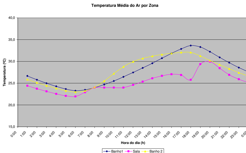
Figura 6.1 – Gráfico da temperatura média do ar por zona (config. atual)
