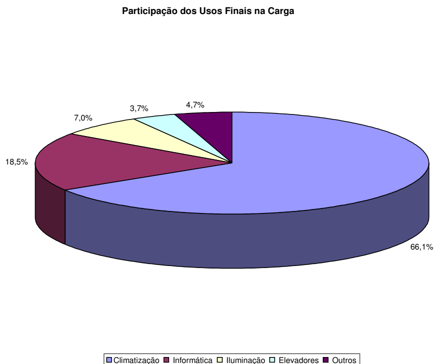
Figura 4.1 – Participação dos usos finais na carga do edifício da Reitoria
