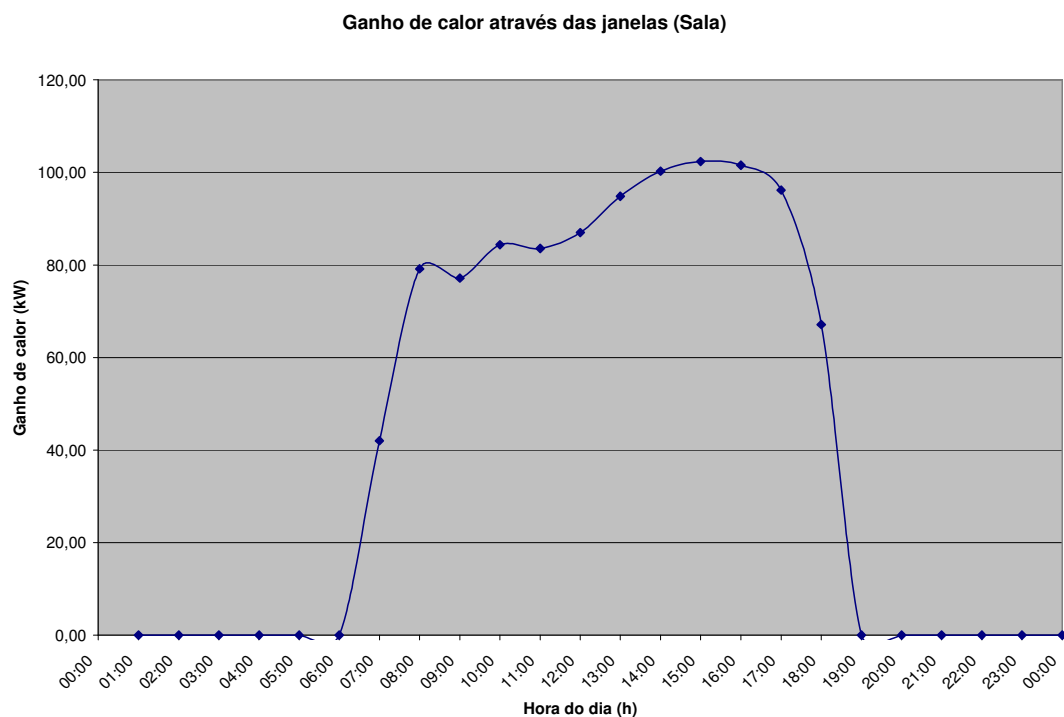
Figura 6.16 – Ganho de calor através das janelas – dia típico de verão (proposta 2)
