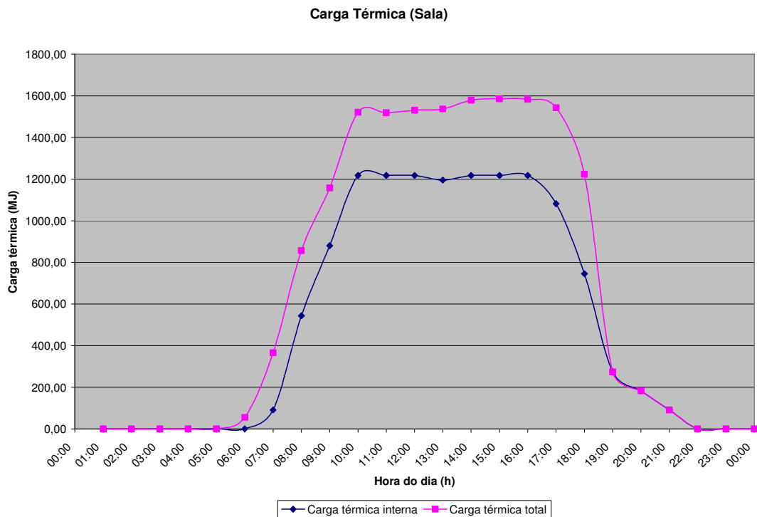
Figura 6.15 – Carga térmica – dia típico de verão (proposta 2)
