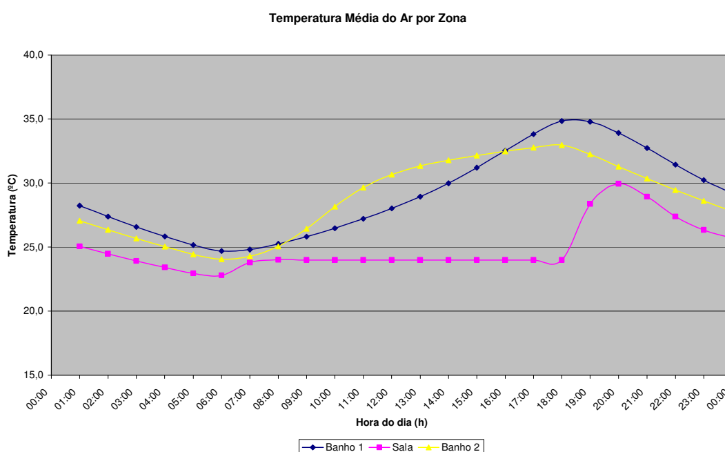
Figura 6.3 – Gráfico da temperatura média do ar por zona (proposta 1)
