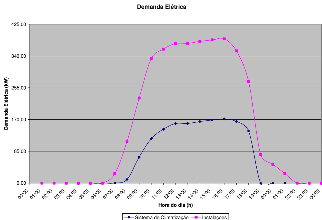
Figura 6.8 – Gráfico da demanda elétrica - dia típico de verão (proposta 3)
