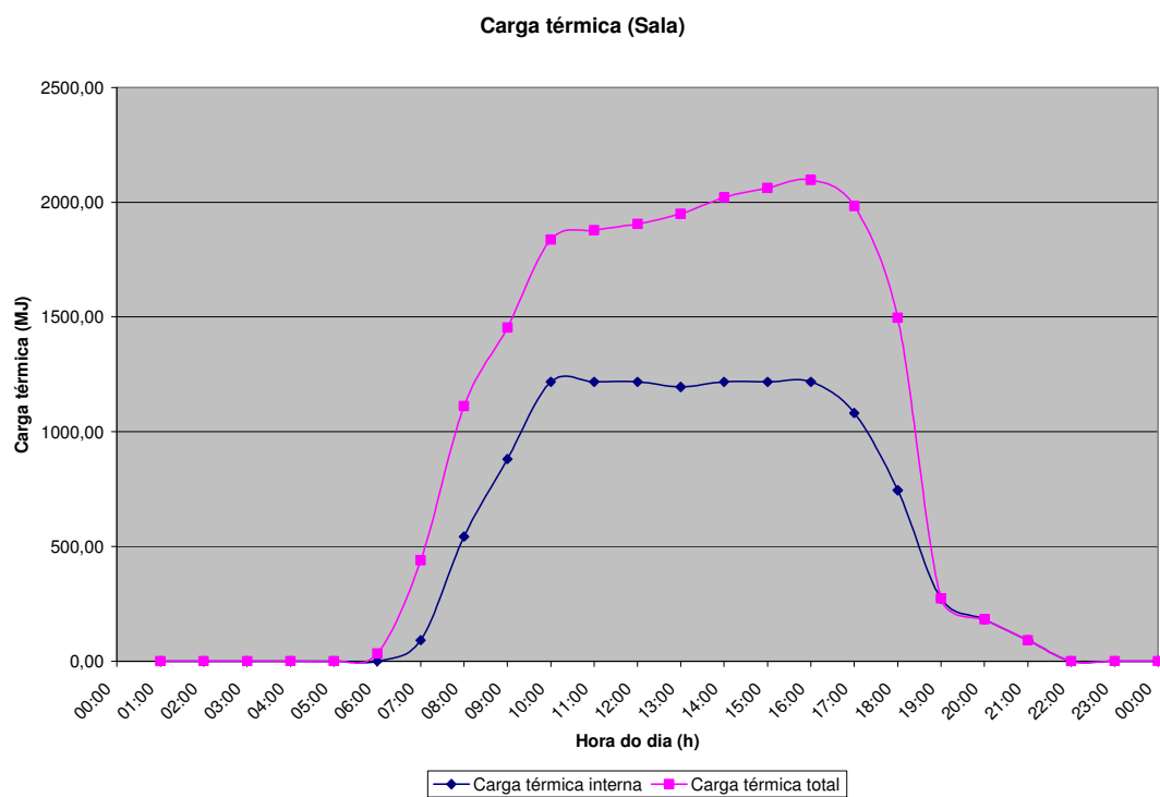
Figura 6.17 – Carga térmica – dia típico de verão (proposta 3)
