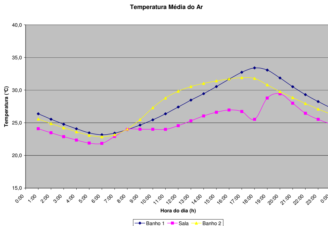
Figura 6.5 – Temperatura média do ar por zona (proposta 2)
