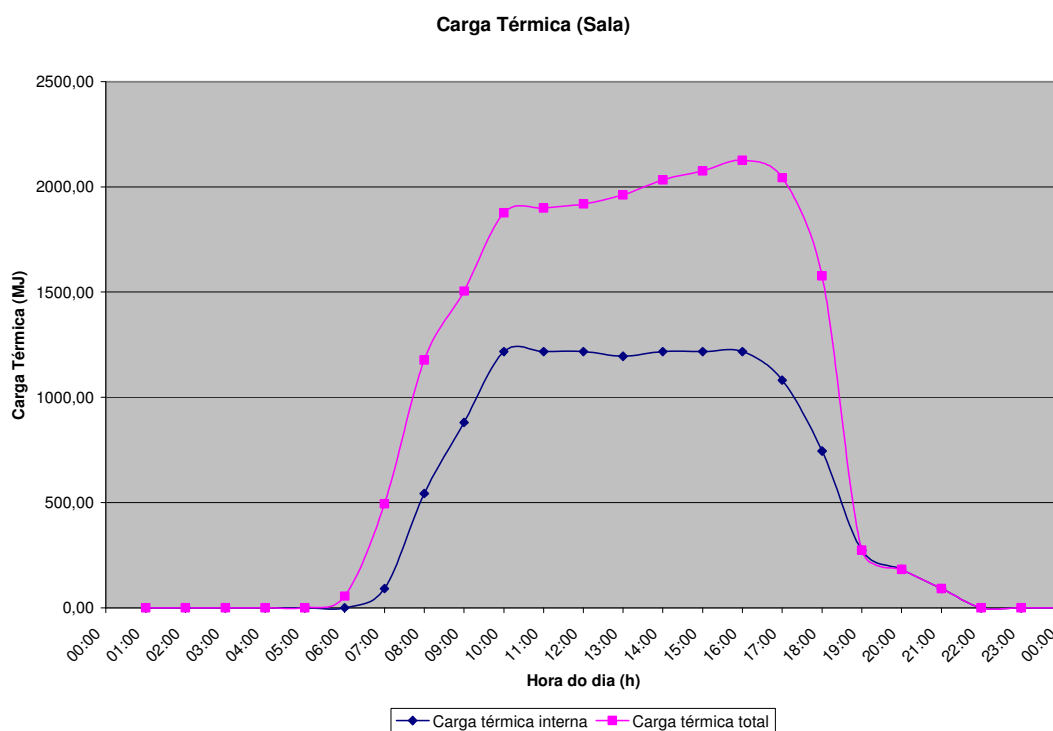
Figura 6.13 – Carga térmica – dia típico de verão (proposta 1)
