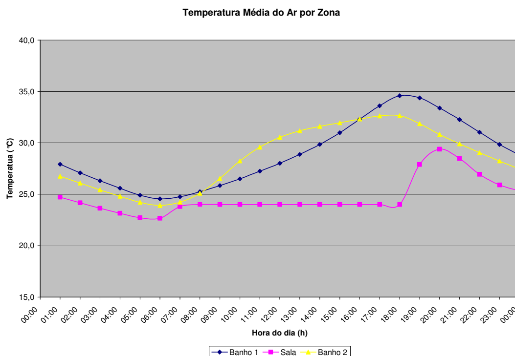
Figura 6.7 – Temperatura média do ar por zona (proposta 3)
