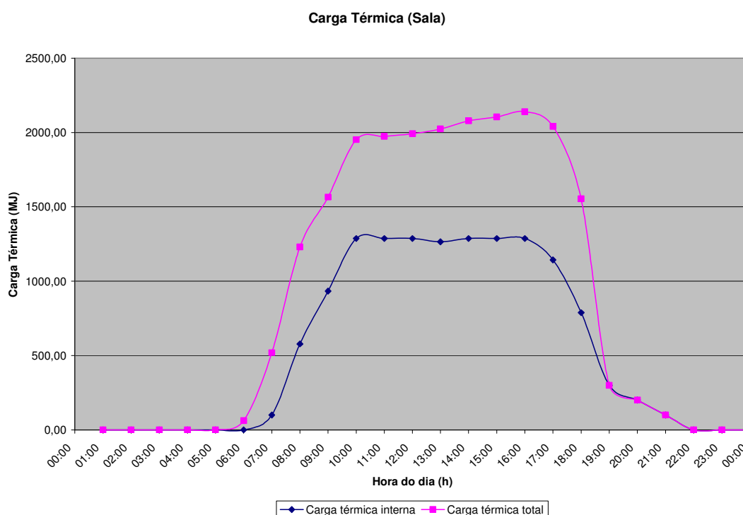
Figura 6.11 – Carga térmica – dia típico de verão (config. atual)
