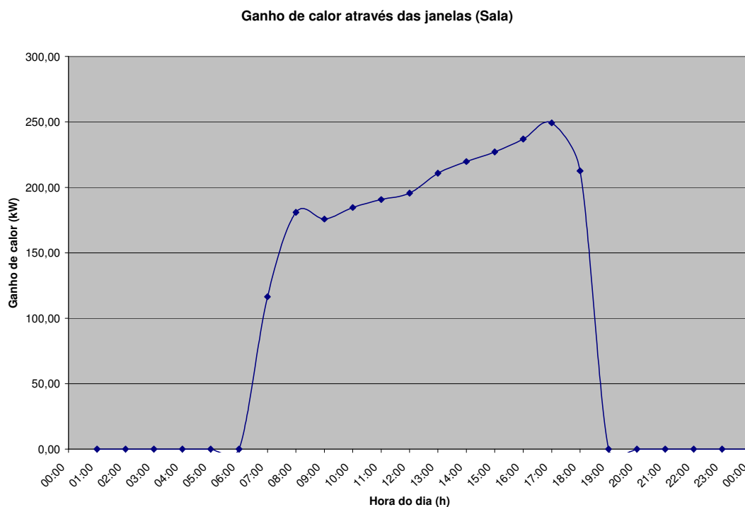
Figura 6.12 – Ganho de calor através das janelas – dia típico de verão (config. atual)
