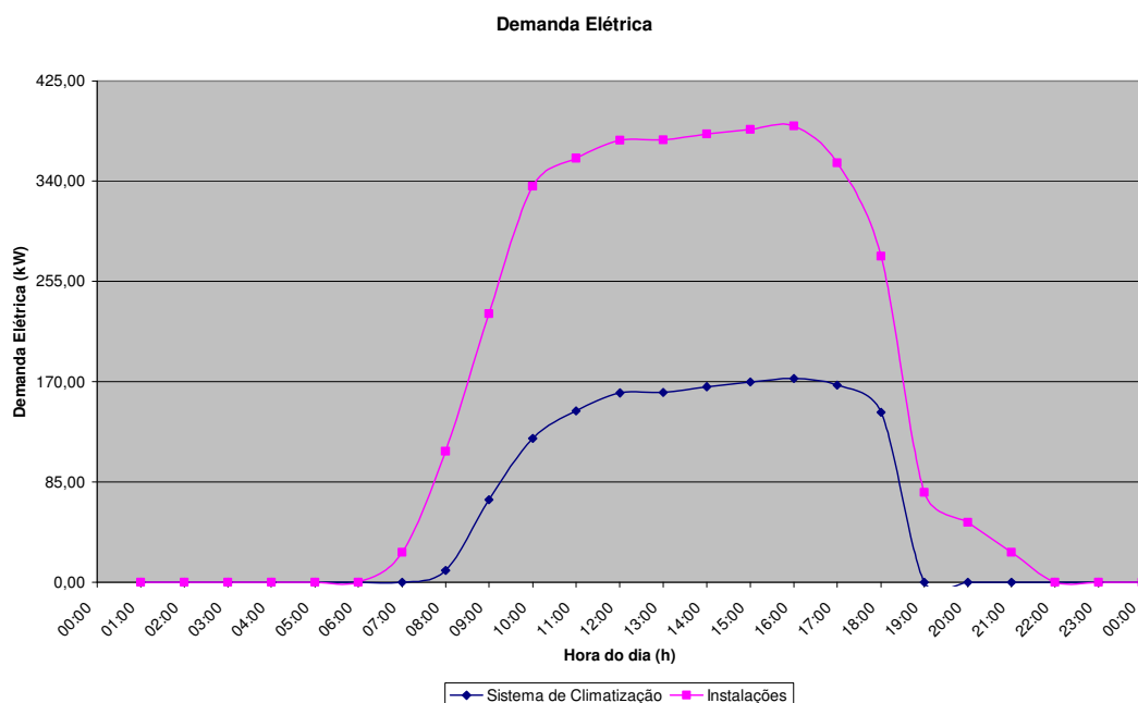
Figura 6.4 – Gráfico da demanda elétrica - dia típico de verão (proposta 1)
