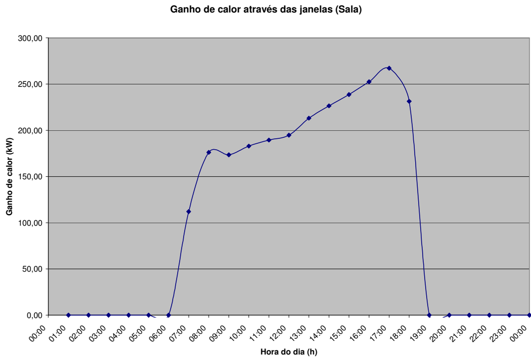
Figura 6.14 – Ganho de calor através das janelas – dia típico de verão (proposta 1)
