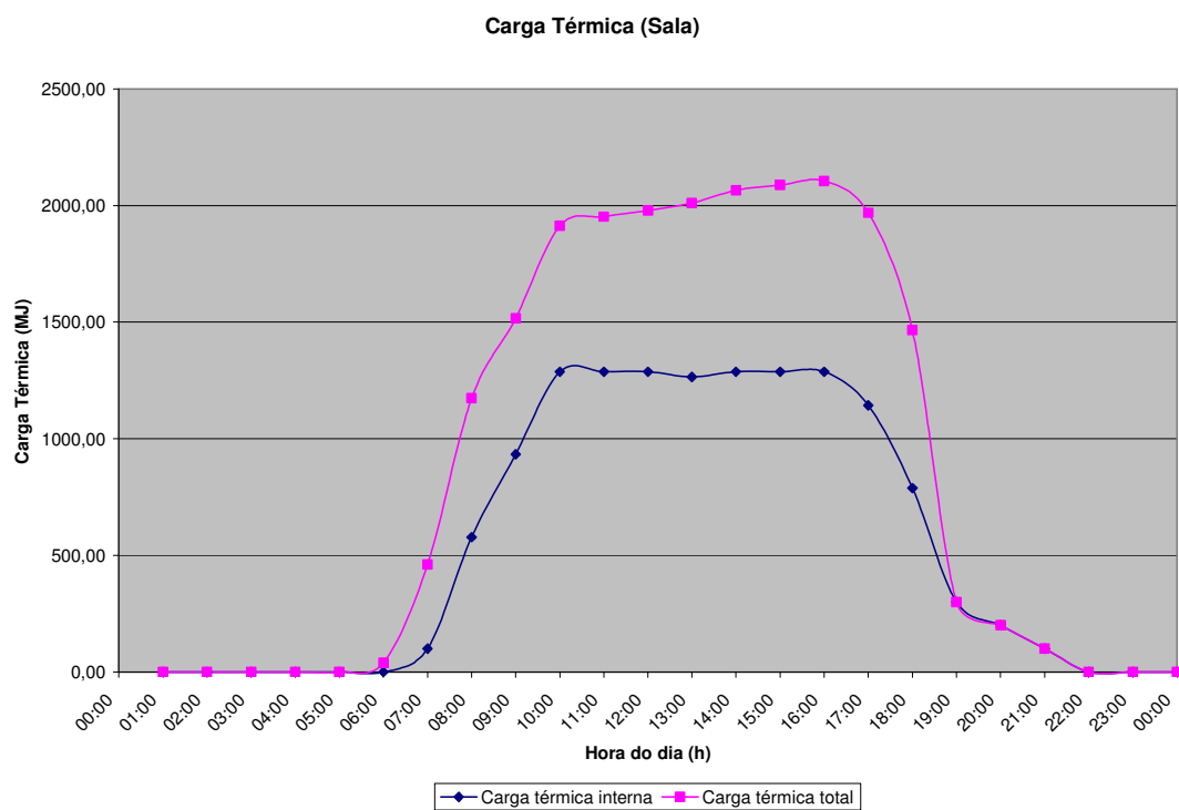
Figura 6.19 – Carga térmica – dia típico de verão (proposta 4)
