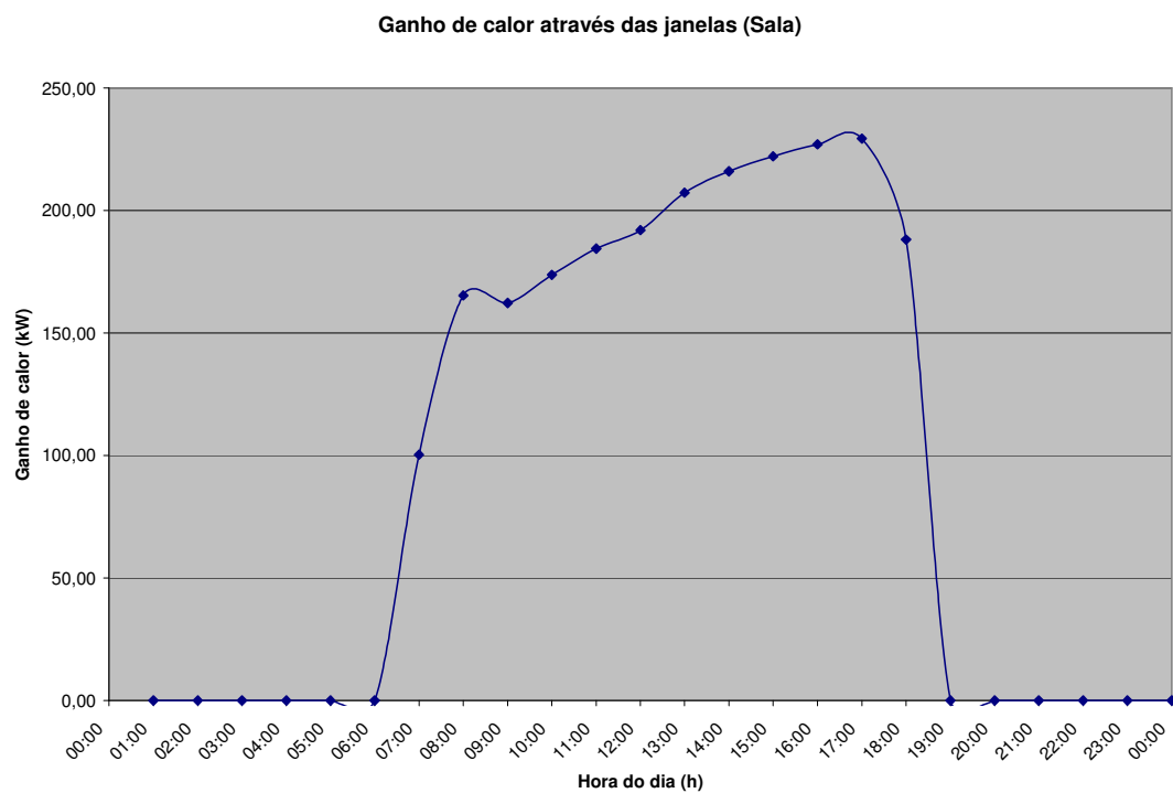
Figura 6.20 – Ganho de calor através das janelas – dia típico de verão (proposta 4)
