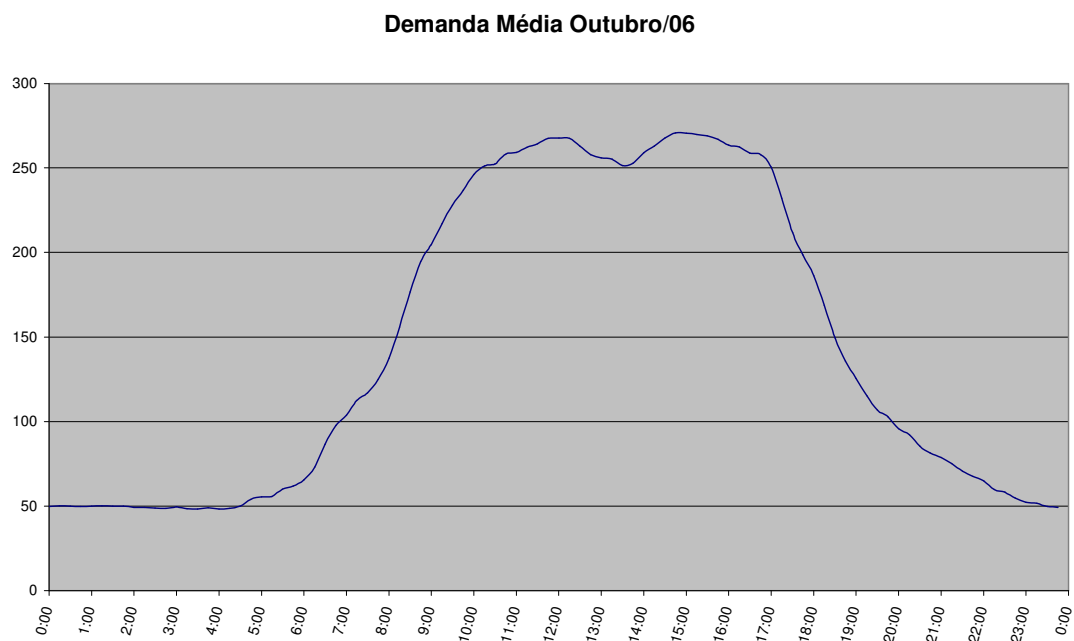
Figura A 10: Demanda média Outubro/2006
