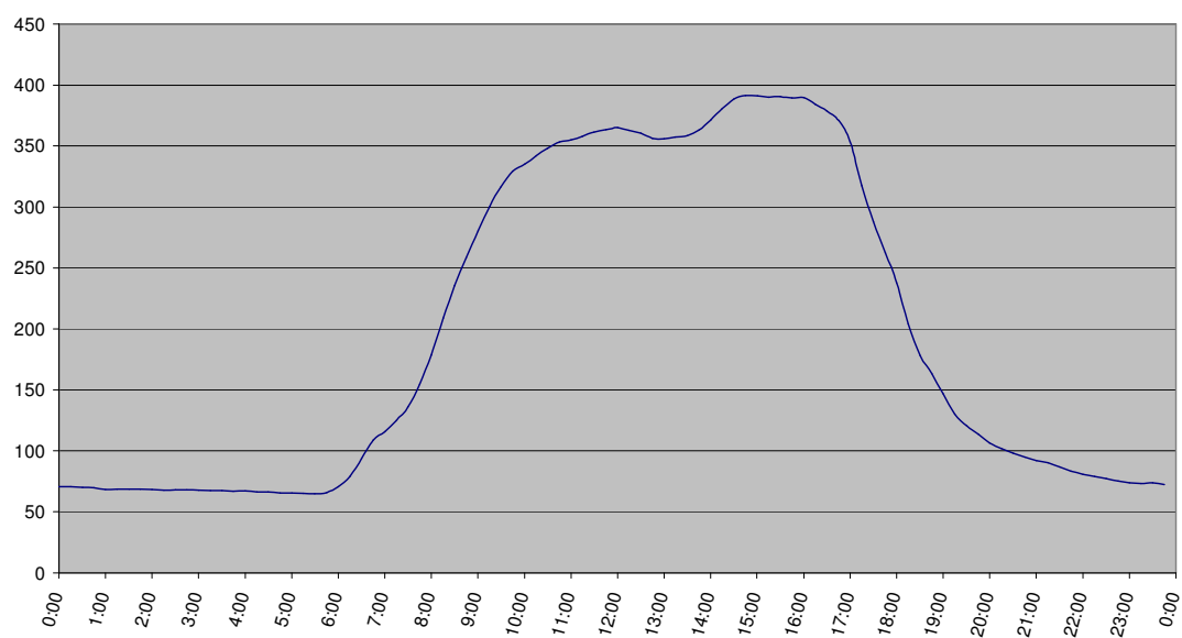
Figura A 3: Demanda média Março/2007
