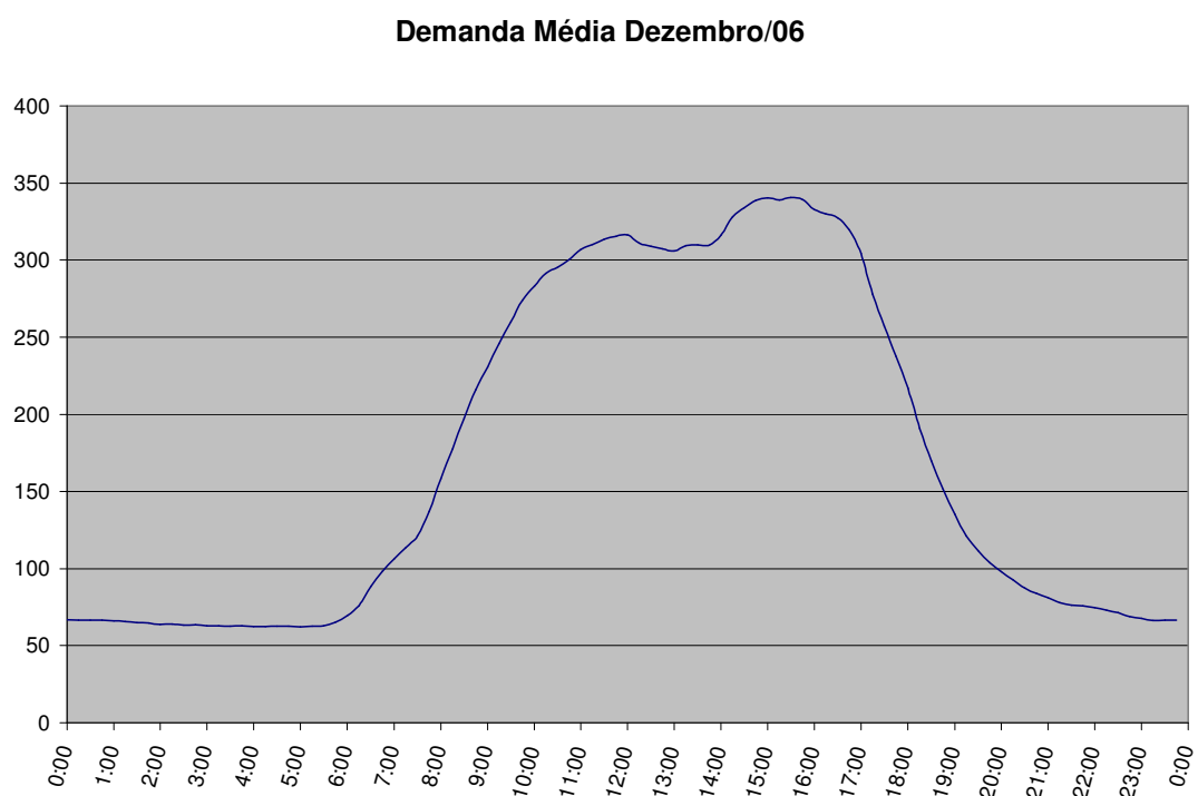
Figura A 12: Demanda média Dezembro/2006
