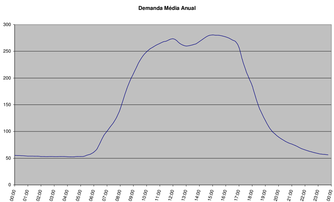
Figura A 13: Demanda média anual
